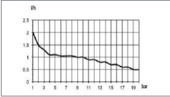
200.5: I/h 0.5 bar 20 Pump head mod. JA
